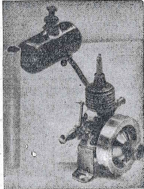
MAŽIAUSIAS PASAULIO MOTORAS New-Yorko išradimų parodoj išstatytas šis motoriuukas. Jis yra lygaus aukštumo kaip cigaretė. Per minutę šis motoriuukas padaro 5.000 apsisukimų
